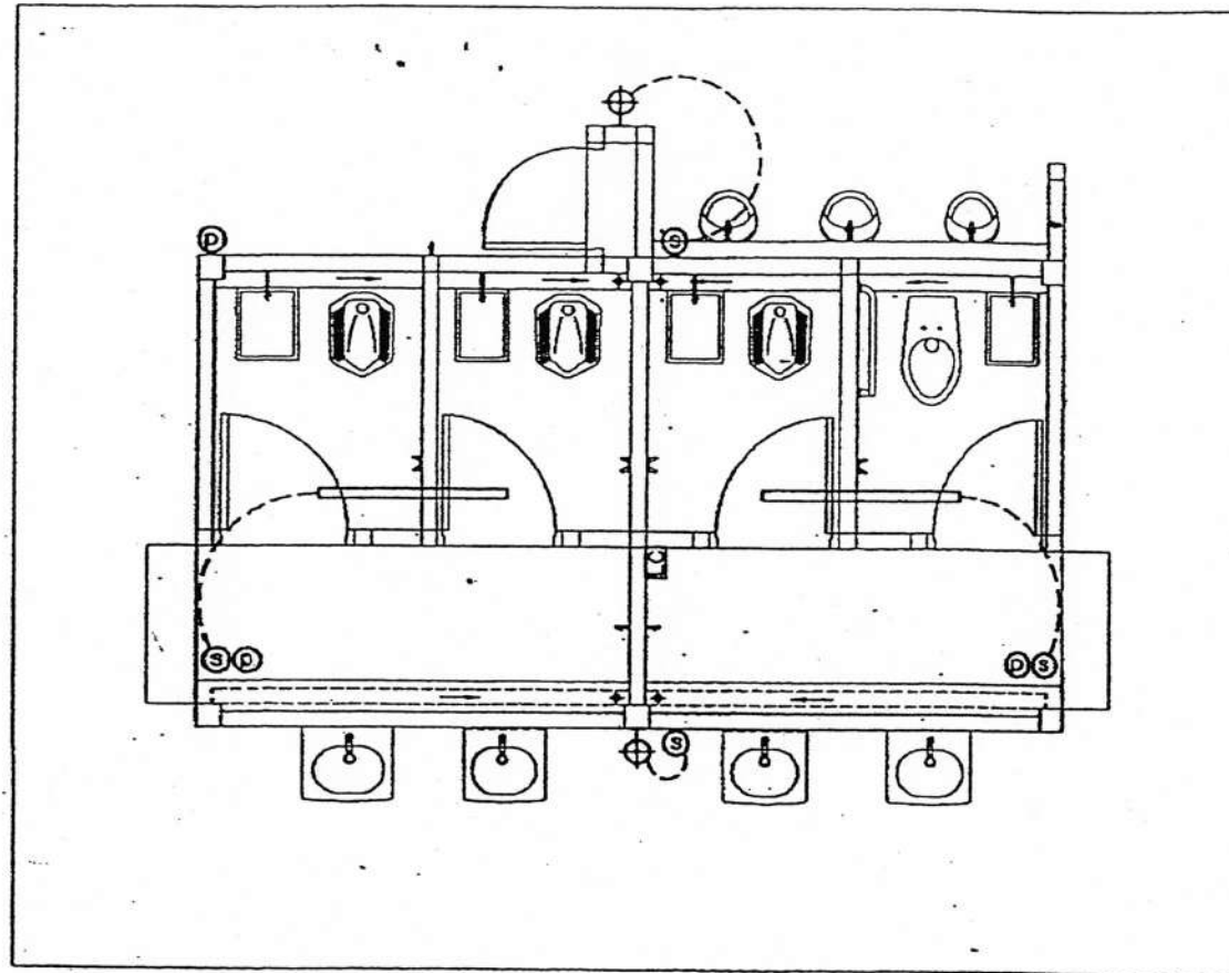
แปลนไฟฟ้า SCALE 1:50
