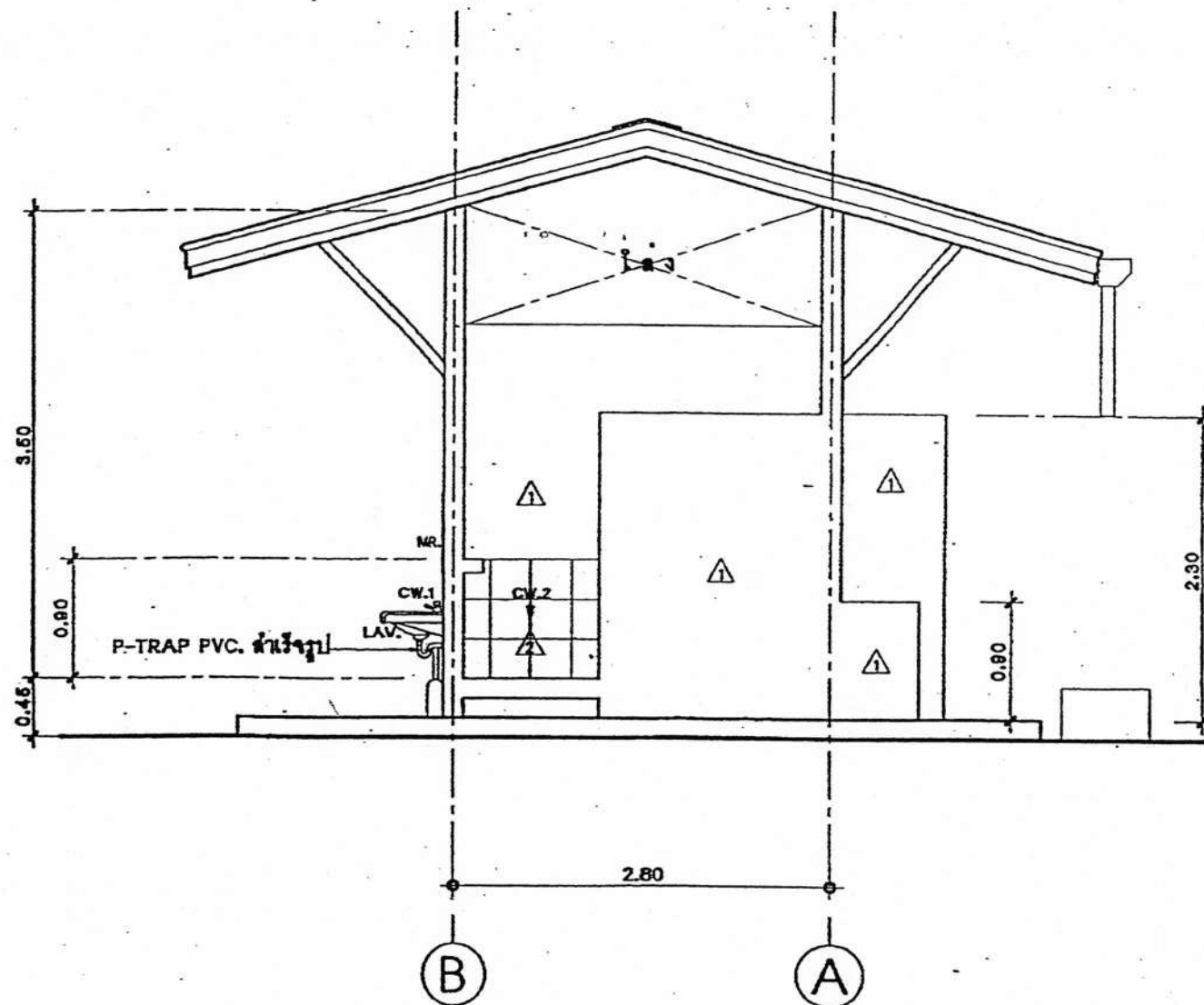
รูปด้าน 2 SCALE 1:50
