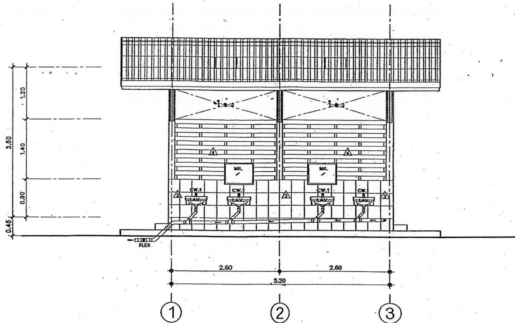
รูปด้าน ① SCALE 1:50
