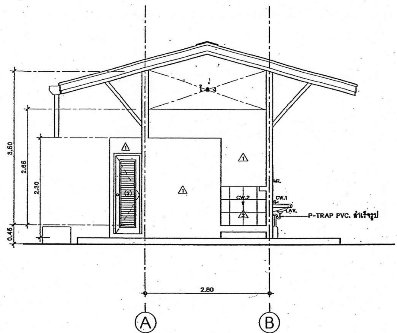
รูปด้าน 3 SCALE 1:50
