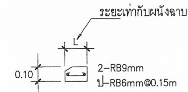
ขยายเอ็นใต้หน้าตั่ง
