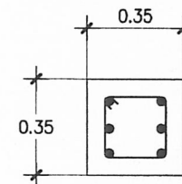
ขยายตอม่อ C1
