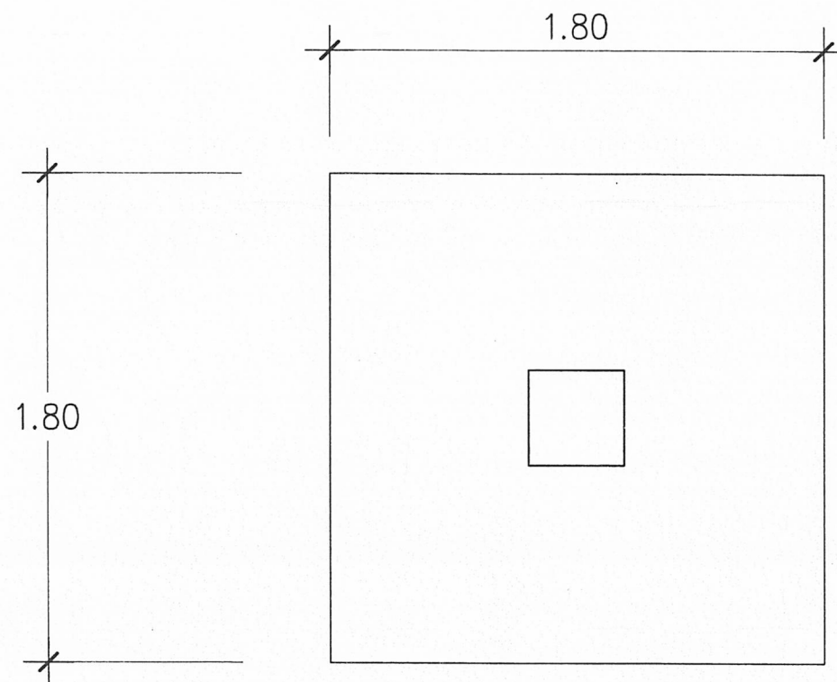
แปลน F1
