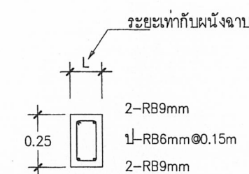
ขยายทับหลังประตู - หน้าตั่ง
