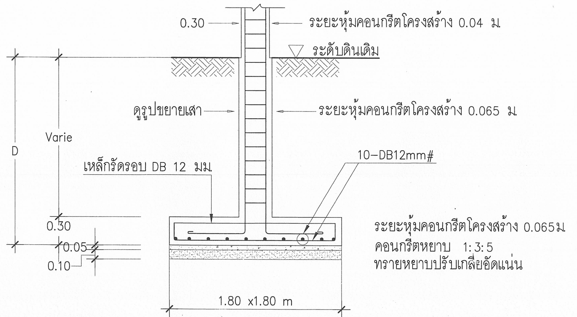
รูปตัด F1
