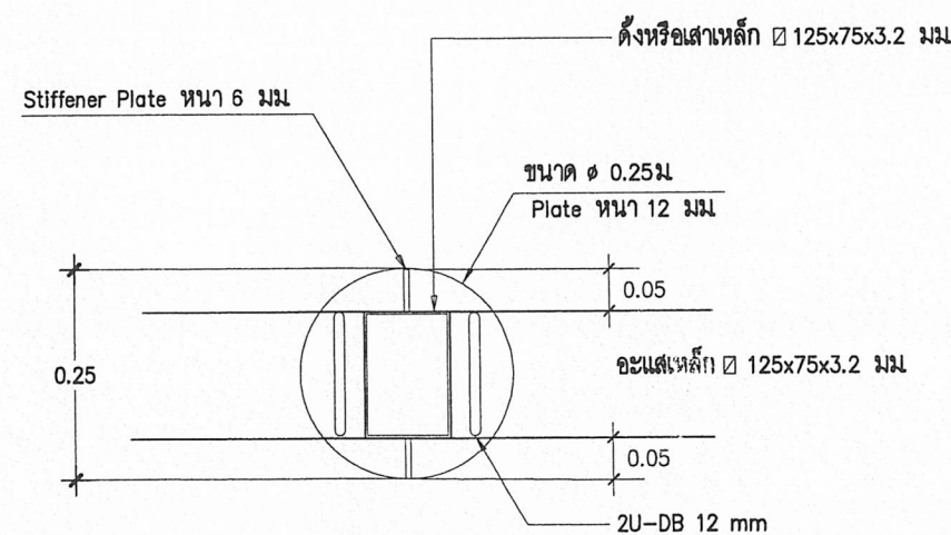
แปลนการยึด CT3 มาตราส่วน 1:10
