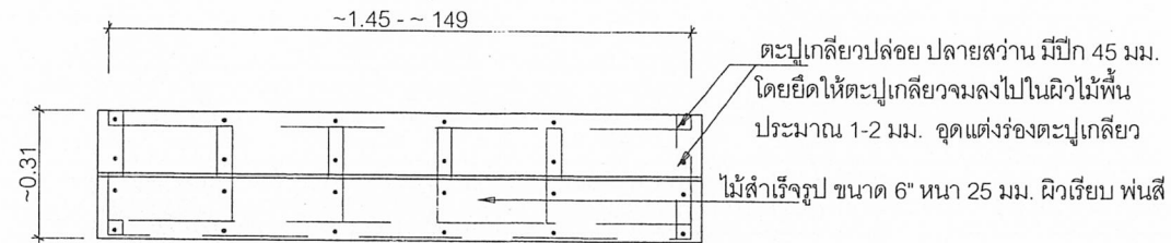
แปลนพื้นเก้าอี้ 1:20
