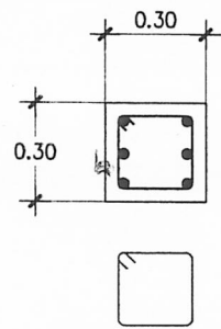
ขยายเสา C1
